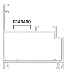
Perfil N° 6040
