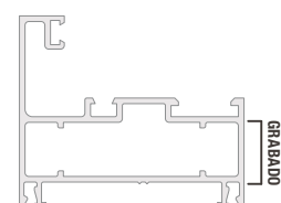
Perfil N° 6059
