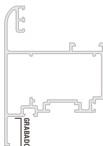
Perfil N° 6056
