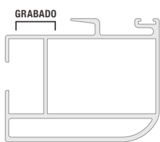
Perfil N° 6035
