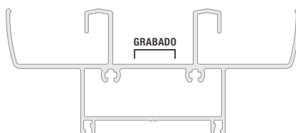
Perfil N° 6037
