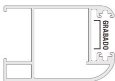
Perfil N° 6071
