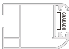
Perfil N° 6034
