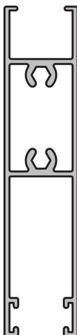
TRAVESAÑO HOJA PUERTA CORREDIZA
