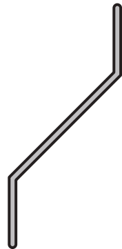
TABLILLA POSTIGON DE 46,6 mm. Perfil: 153 Peso: 0,186 Kg/m Matriz: M2009
