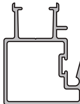
PARANTE CENTRAL REFORZADO HOJA
