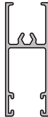
ZOCALO Y CABEZAL - HOJA CORREDIZA
